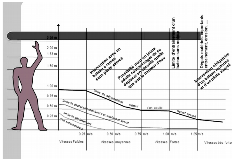
Figure 22 : Mobilité en terrain inondé en fonction de la vitesse et de la hauteur d'eau
